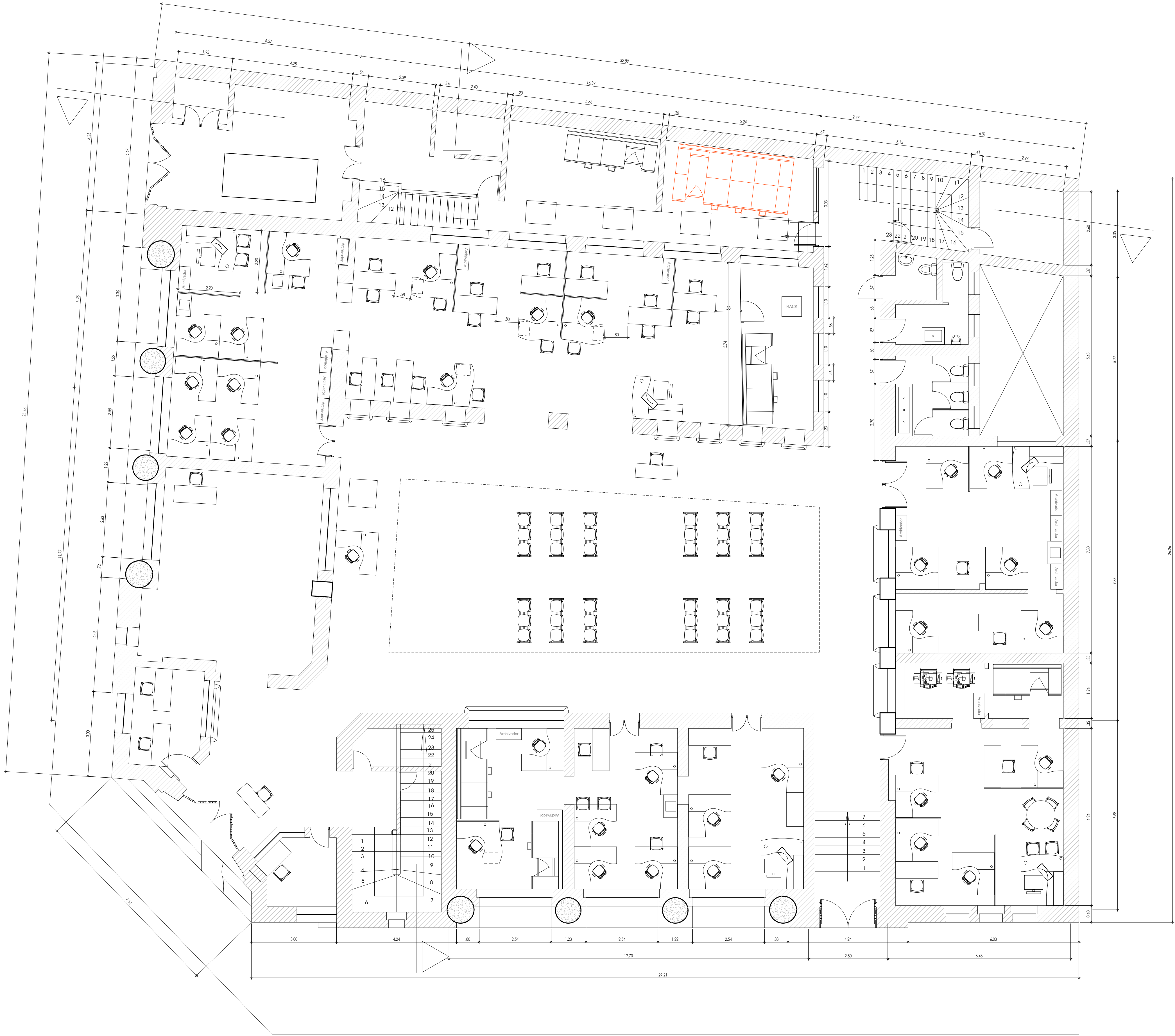
1 PLANTA PRIMER PISO ESTADO ACTUAL ESCALA 1 : 75
