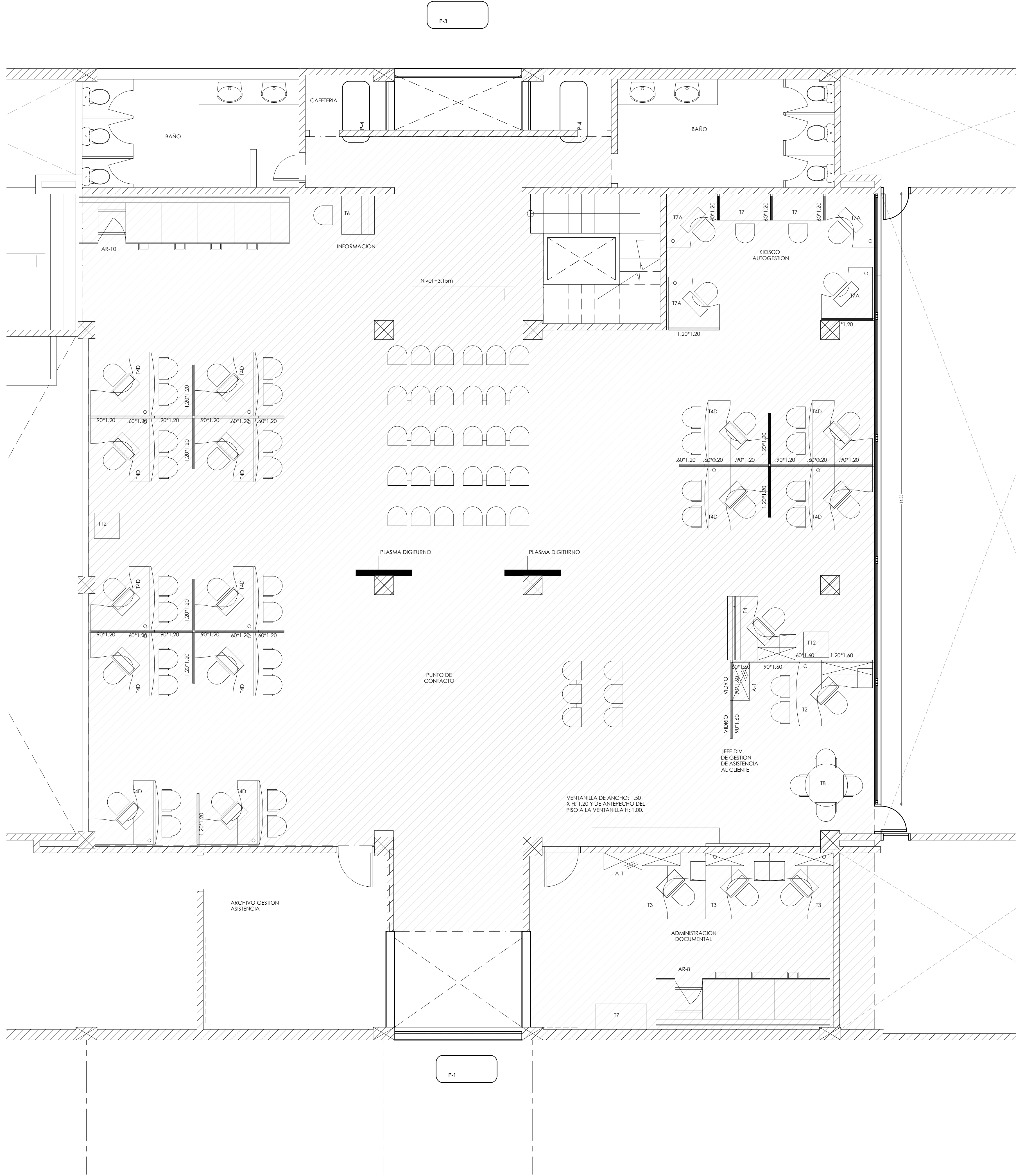
1 PLANTA SEGUNDO PISO ESTADO ACTUAL
