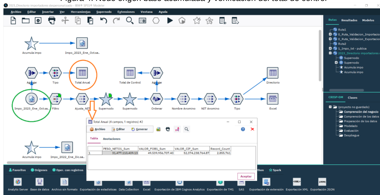
Figura 4. Nodo origen base acumulada y verificación del total de control
